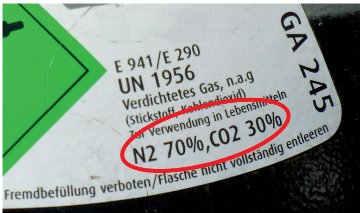
Abb. 2: Beschriftung einer Druckgasflasche mit Mischgas mit 70 % \text{N}_2 und 30 % \text{CO}_2 -Anteil
